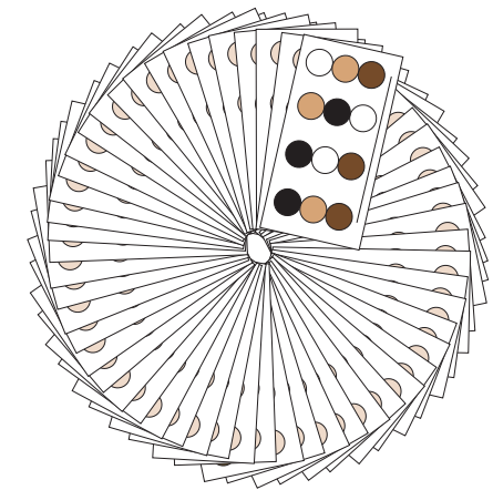
課題カード
